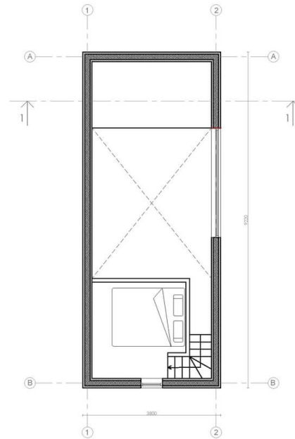
Loft Plan
